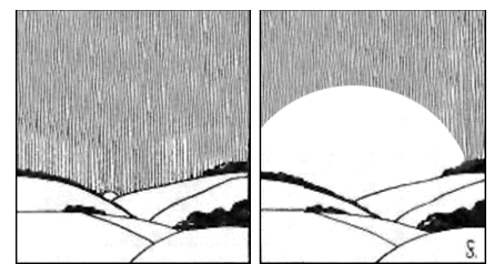
Abb. 4. Der Tertiärmond vor Sinflutbeginn links in Hirsekorngröße der heutige Mond zum Vergleich der Größenverhältnisse.
