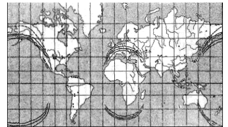
Abb. 3. Die Flutberge zur Zeit des eintägigen Monats.
