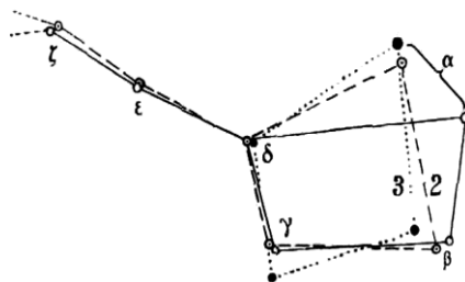
Abb. 85. Sternbild Großer Bär vor 60 000 Jahren.
