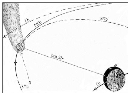
Abb. 52. Der Einfang des Mondes Luna und der Untergang von Atlantis.
