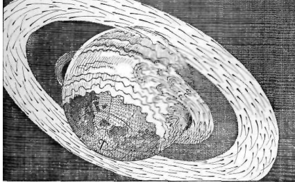
Abb. 5. Die beginnende Sintflut. Die Auflösung des Mondes Dhöbus und der Einsturz auf die Erde.
